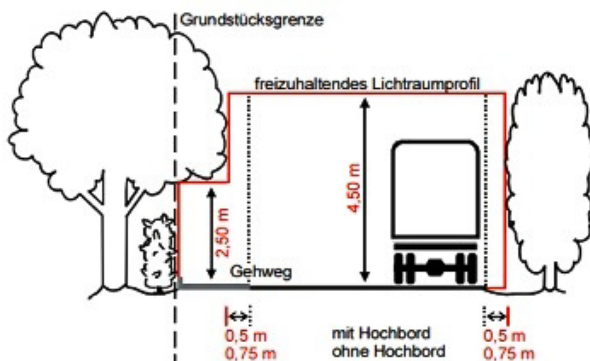
Skizze Lichtraumprofil, Foto: (Quelle: https://www.buergerinitiative-tunzenberg.de/fa_abstand_halten.html )
